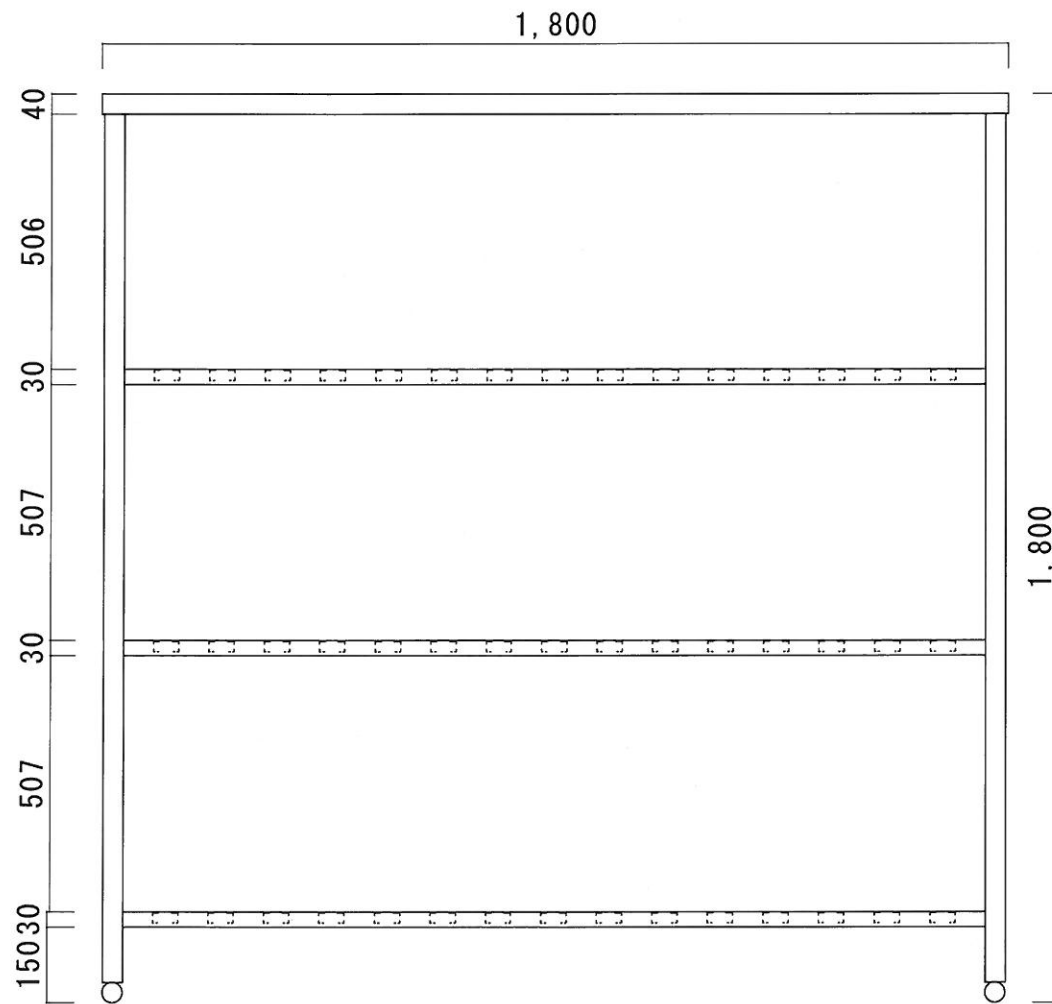
正面図
