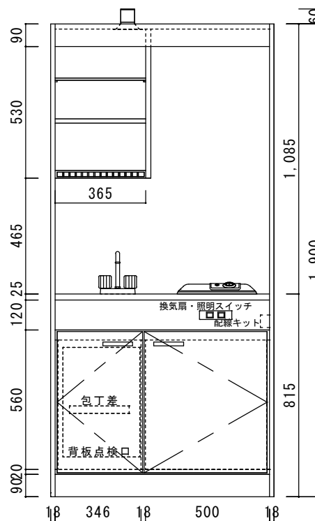
正面小口カバー取付後W=902
